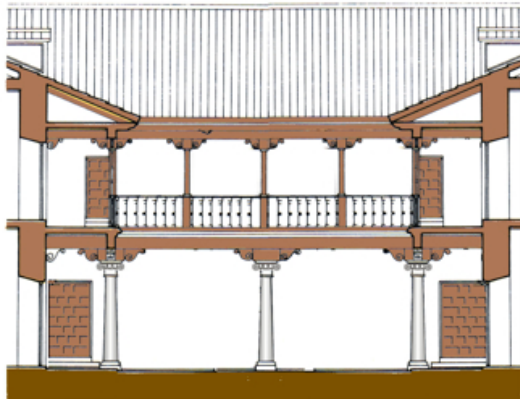
6. Alzado del patio
